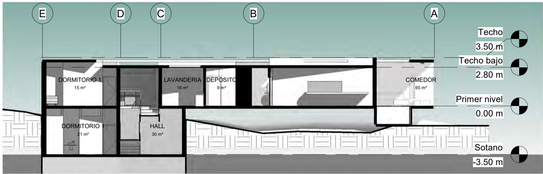
1 CORTE A-A 1 : 150
