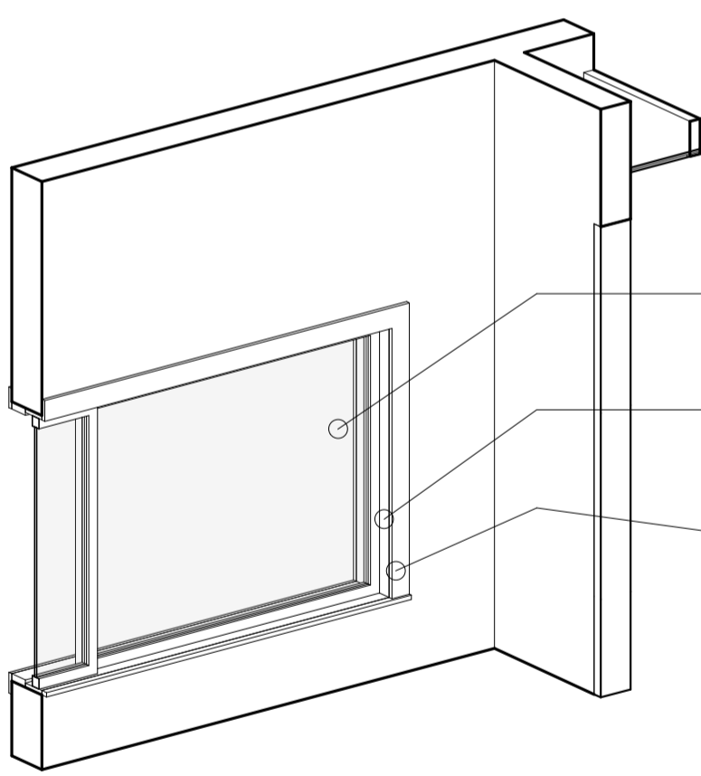
2 DETALLE DE VENTANA
